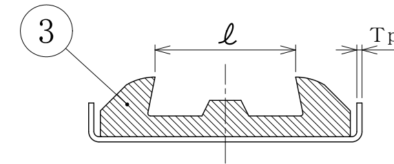
A-A断面詳細図
