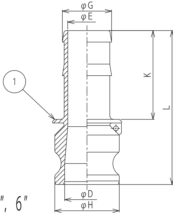
633-E SST サイズ別寸法表 (単位: mm)
