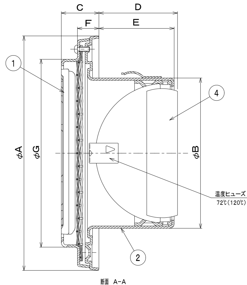
断面 A-A
