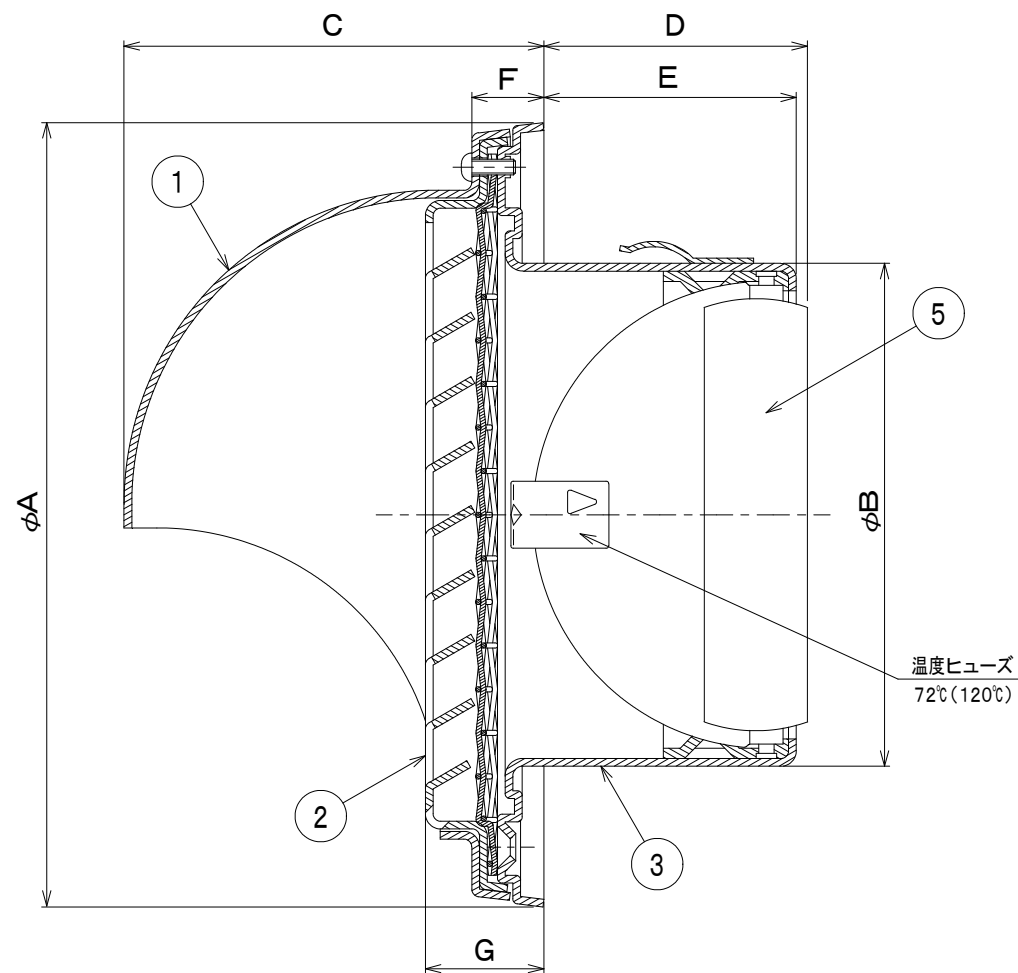
断面 A-A
