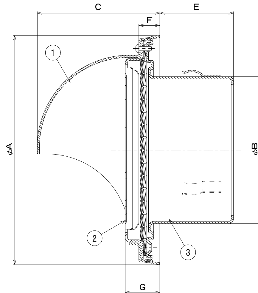
断面 A-A
