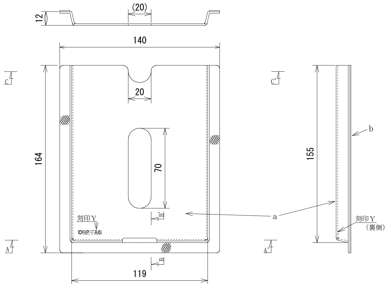
C－C' 矢視図
