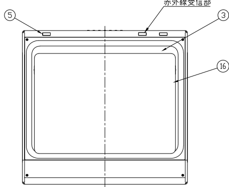
底面図
