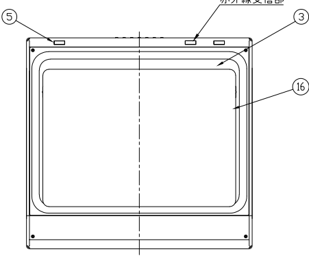
底面図
