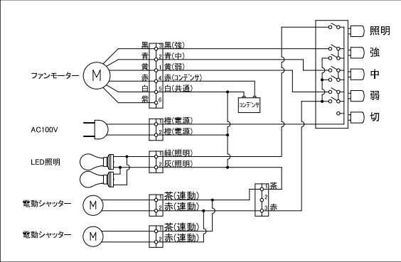
□結線図
