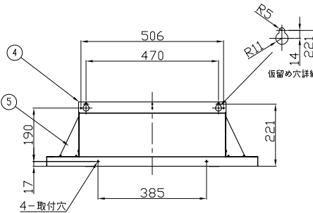
背面取付図
