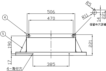
背面取付図
